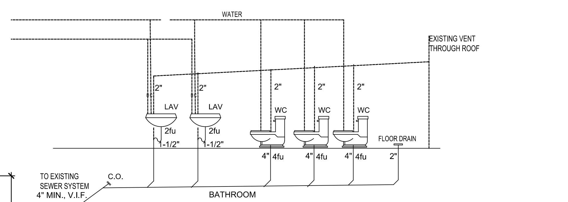
4 PLUMBING RISER DIAGRAM SCALE: N.T.S.
